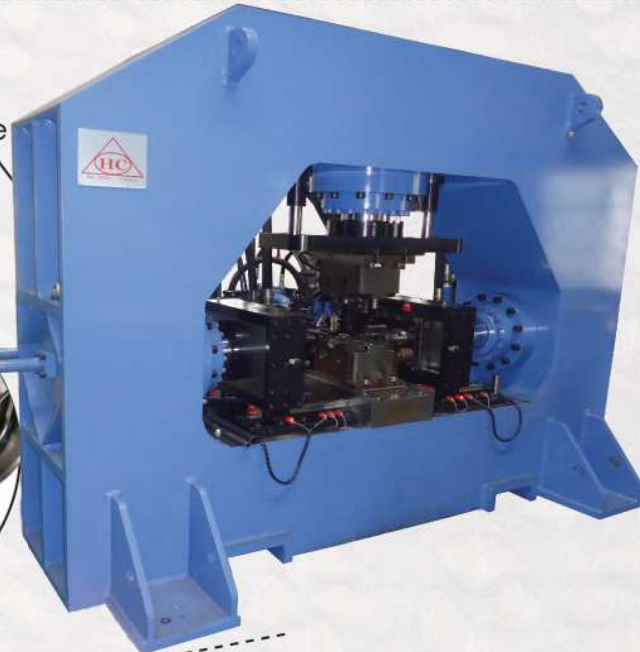
車頭管擴管機 Head pipe / Head tube
