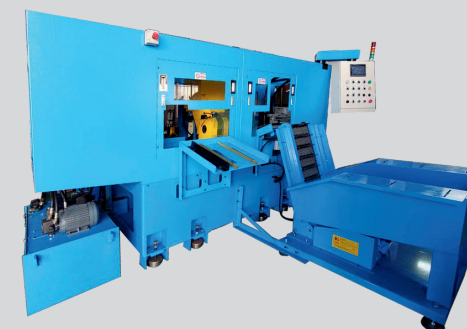
2 Ways Cut & Chamfer Machine HC8003 自動伺服雙端切斷倒角機 Fork pipe/ Shock absorbers
